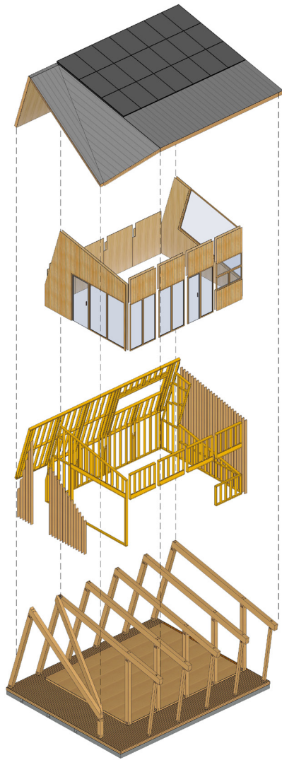
园林学院风景建筑研究中心与材料学院木结构建筑设计中心联合教学与合作设计的近零能耗混合式木结构建筑——中林低碳驿站于北林校园内建成。
