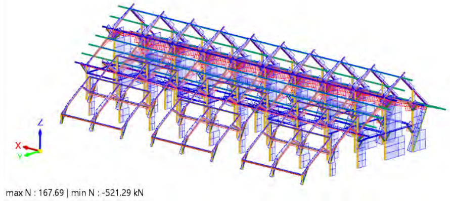
轴力N分布图
