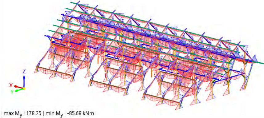
弯矩My分布图
