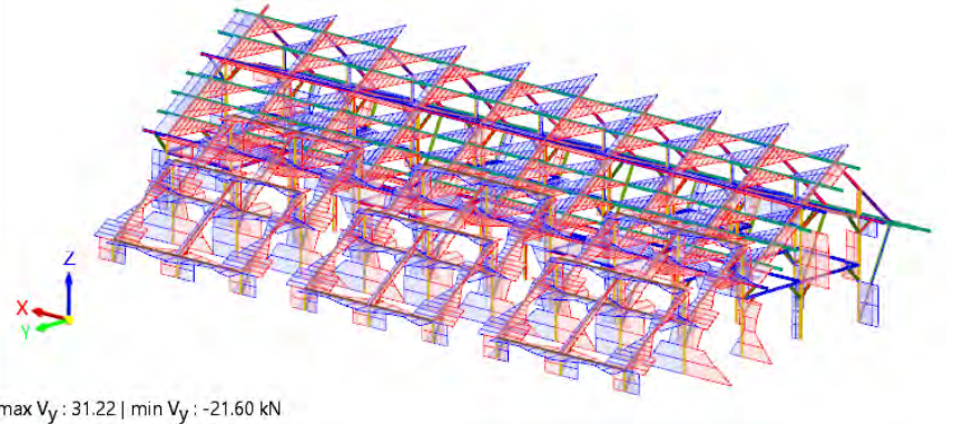
剪力Vy分布图
