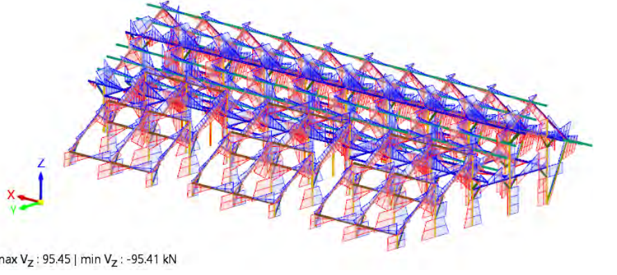
剪力Vz分布图
